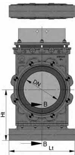
Стандартное исполнение
