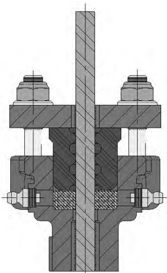
Секция F-F
