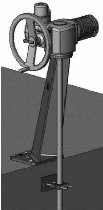
Наклонная колонна
