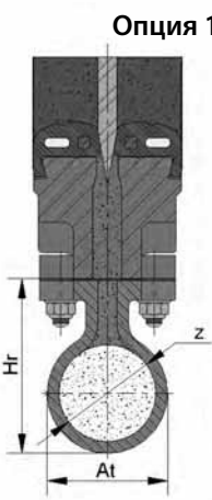
Секция B-B
