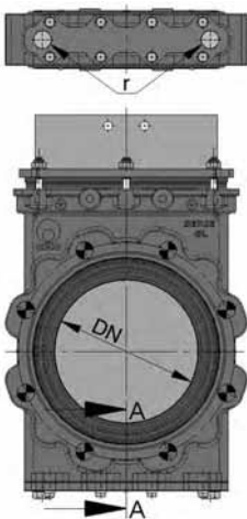
Стандартное исполнение
